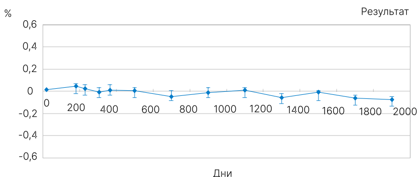
Тест на изменение размеров в течение 5 лет эксплуатации
